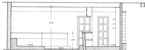
SECCION LONGITUDI
