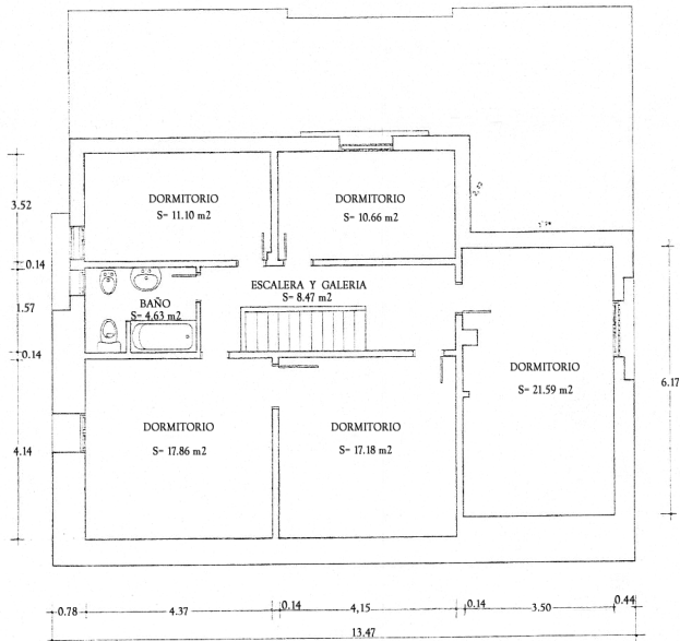
PLANTA ALTA
